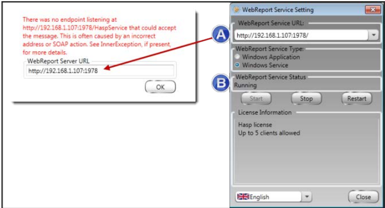
Figura 26 – URL e configurações do serviço WebReport
