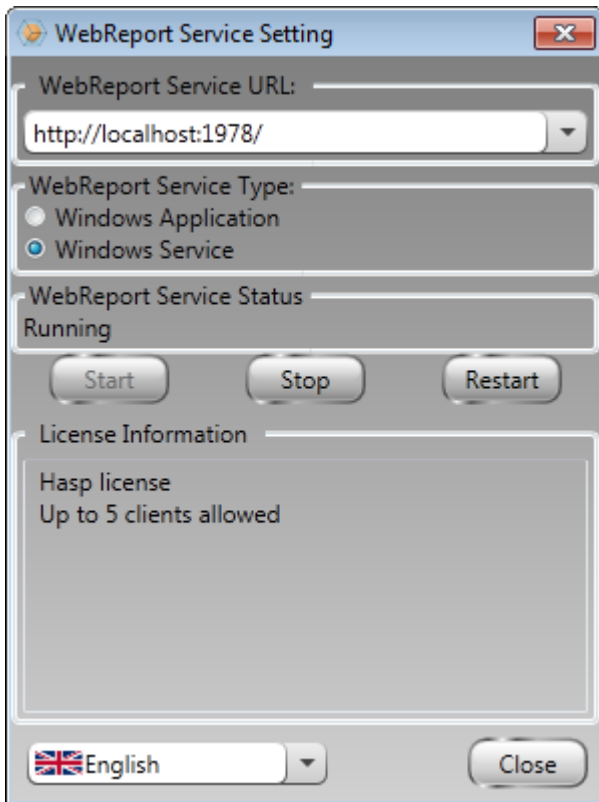
Figura 12 –Utilitário da configuração do serviço WebReport
